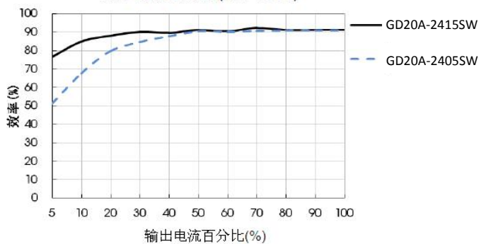
效率/输出负载(Vin=24V)
