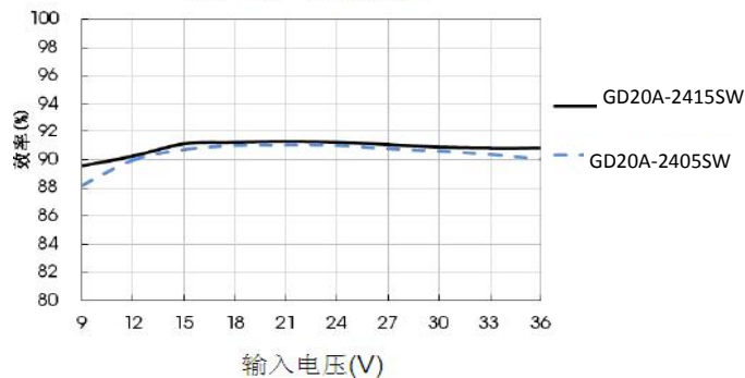
效率/输入电压(满载)
