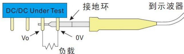
图 2-4 示波器靠测法
