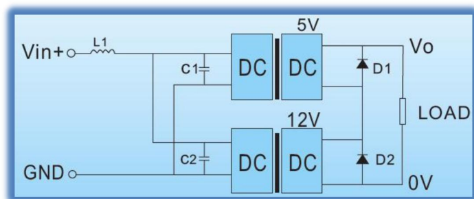
图 3-1 模块的串联应用接法 1
