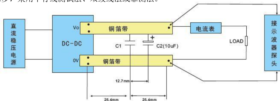
图 2-2 平行线测试法
