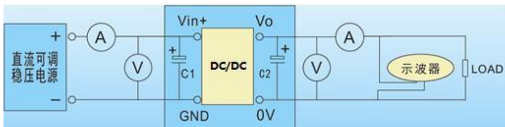
图 2-1 开尔文测试法
