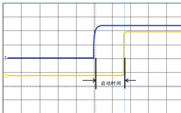
图 2-6 启动时间测试
