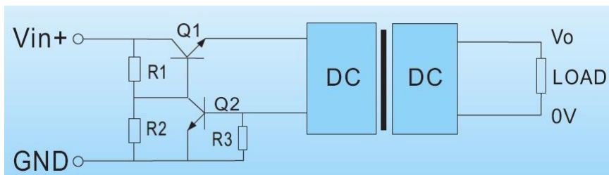
图 3-10 持续过流保护电路。
