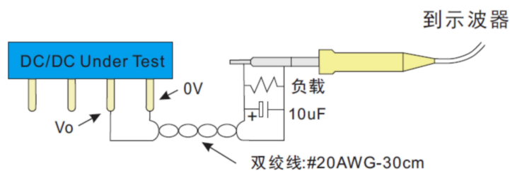
图 2-3 双绞线测试法
